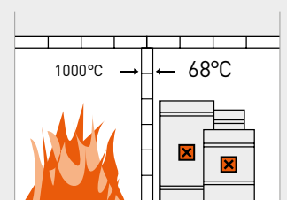
Ytong akytasis betonas sienos storis 150 mm
