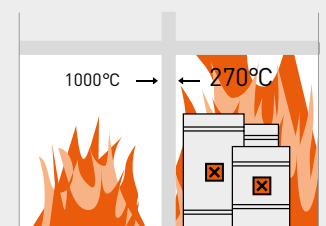
Paprastas betonas sienos storis 150 mm
